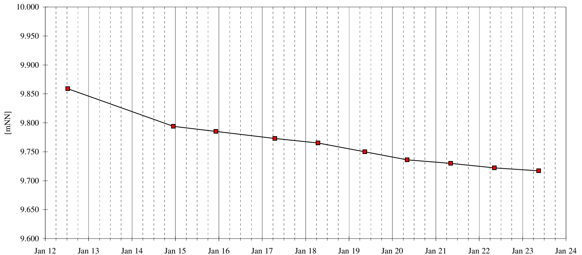
Setzungskurve
