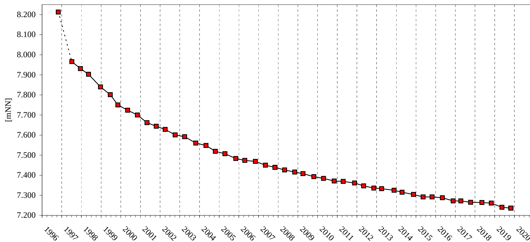
Setzungskurve
